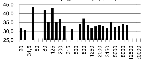
Schalldruckpegelkurve [dB(A) zu Hz] 5)
